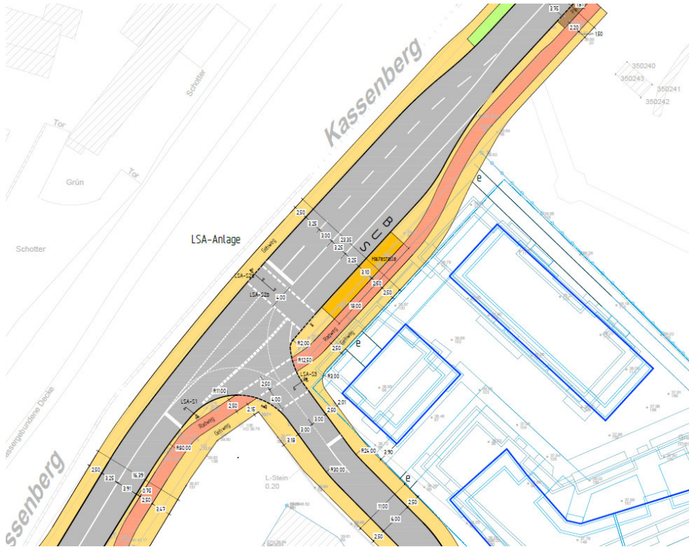
Abb. 3: geplanter Kreuzungsumbau Kassenberg/ Planstraße (Verkehrerschließungsplanung Lindgensareal Vorplanung (Endfassung), büro stadtVerkehr, Hilden, 29.06.2022)
